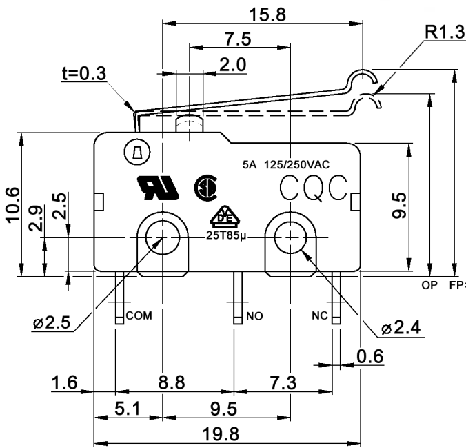
Actuator 04
