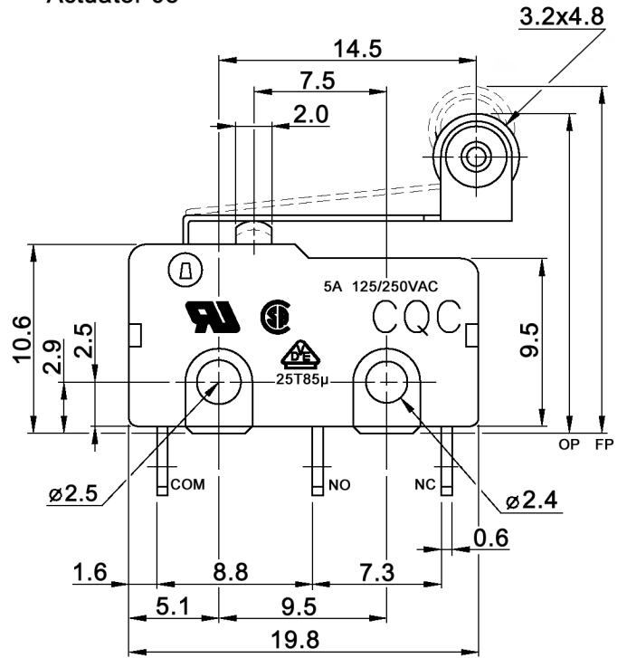
Actuator 05
