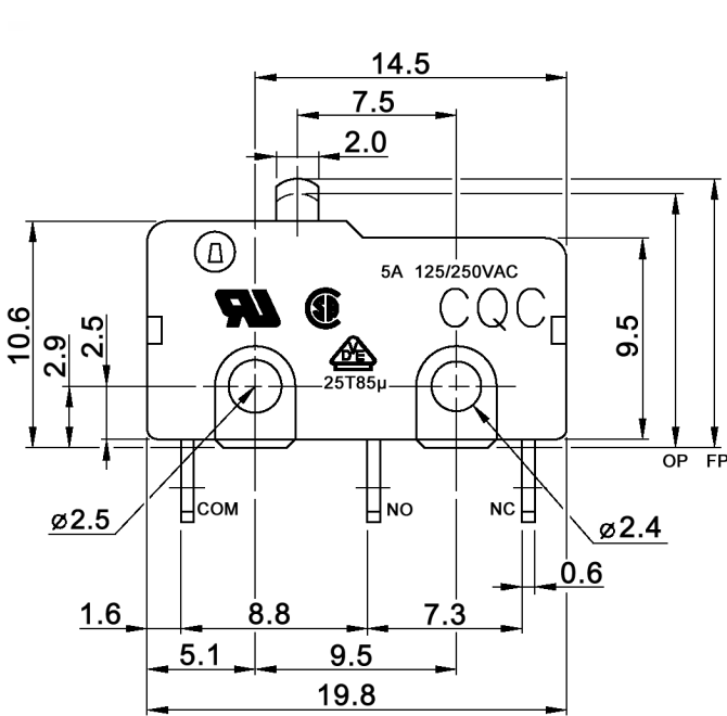
Actuator 00
