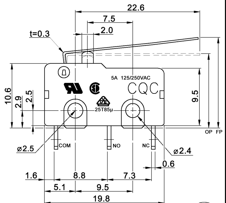
Actuator 03
