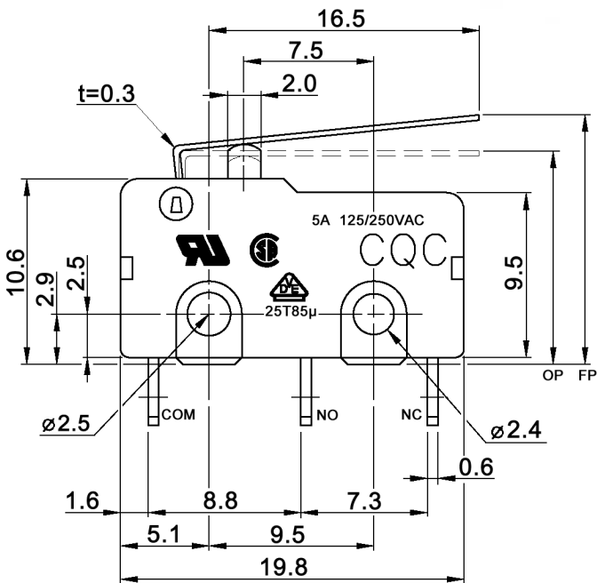
Actuator 02
