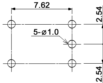
P.C. LAYOUT
